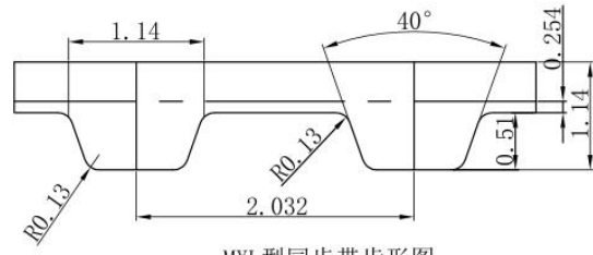
MXL型同步带齿形图
