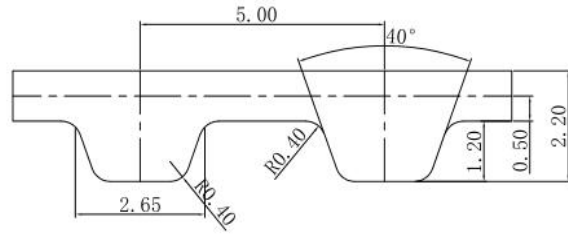
T5型同步带齿形图
