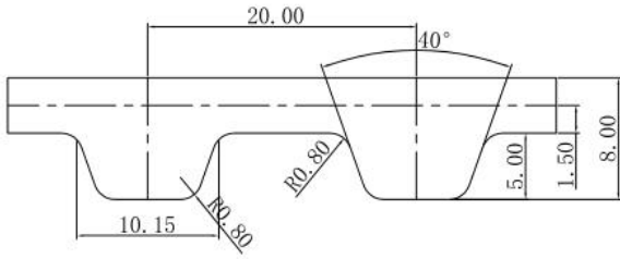
T20型同步带齿形图
