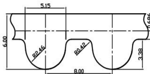
8M带齿形图
